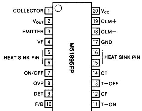
Outline 20P2N-A
